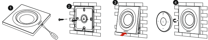
Kyttimein seinäasennus / Vägmontering av strömbrytare / Switch Wall Mounting
