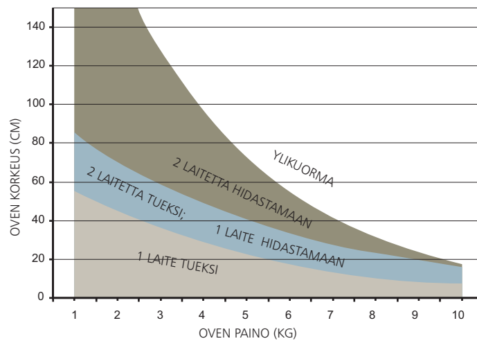
MITOITUS 90° YLÖSAUKEAVALLE OVELLE
