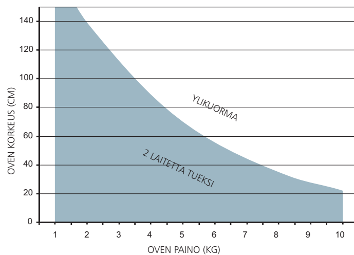
MITOITUS 90° ALASAUKEAVALLE OVELLE
