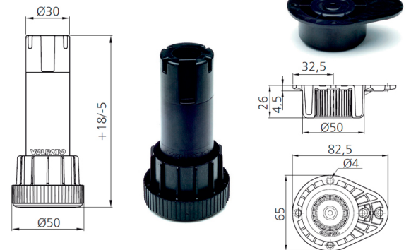
Ruuvikiinnitteinen sokkelijalka
