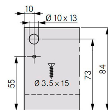
Takasarjan asennusmitat
