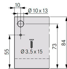
Takasarjan asennusmitat
