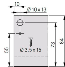
Takasarjan asennusmitat
