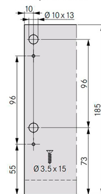
Takasarjan asennusmitat
