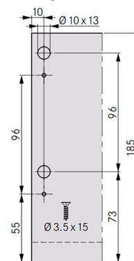
Takasarjan asennusmitat
