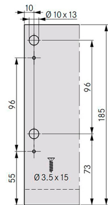
Takasarjan asennusmitat
