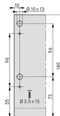
Takasarjan asennusmitat
